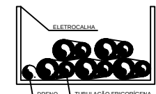
DETALHE 8 - PASSAGEM DE LINHAS PELA ELETROCALHA SEM ESCALA
