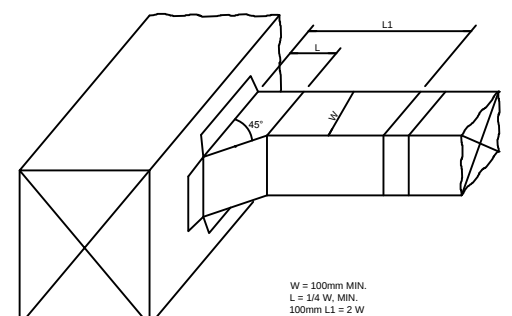
CONEXÃO PARA RAMAL COM DUTO RETÂNGULAR SEM ESCALA
