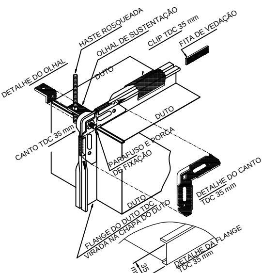
DETALHE - ACESSÓRIO DE FIXAÇÃO SEM ESCALA
